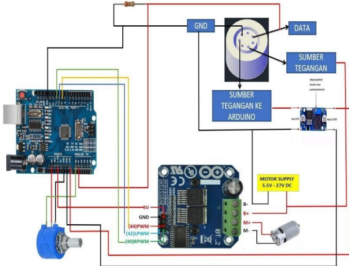
Gambar 2 Desain Elektrikal
