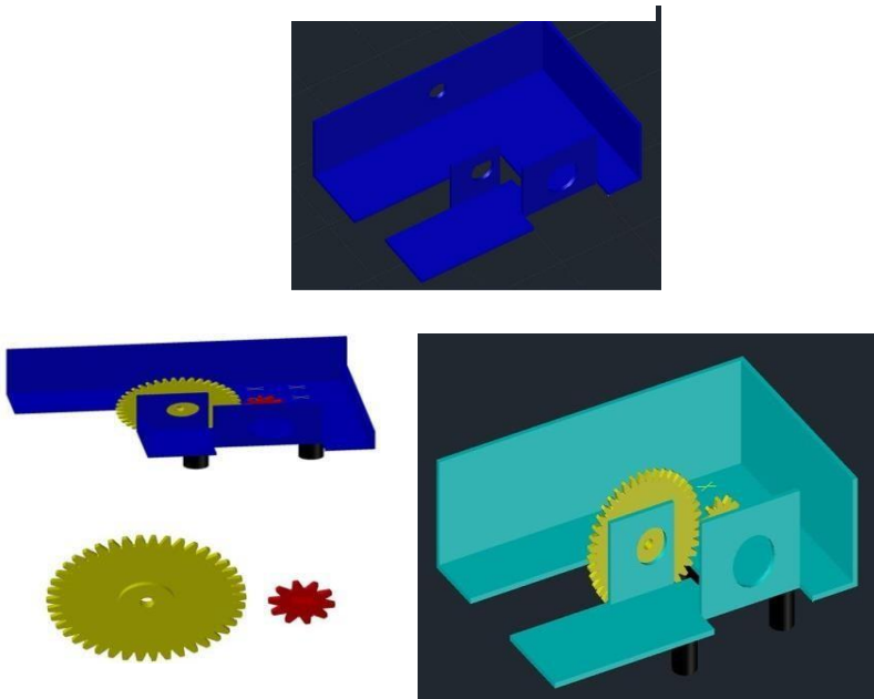
Gambar 4 Desain Mekanikal
