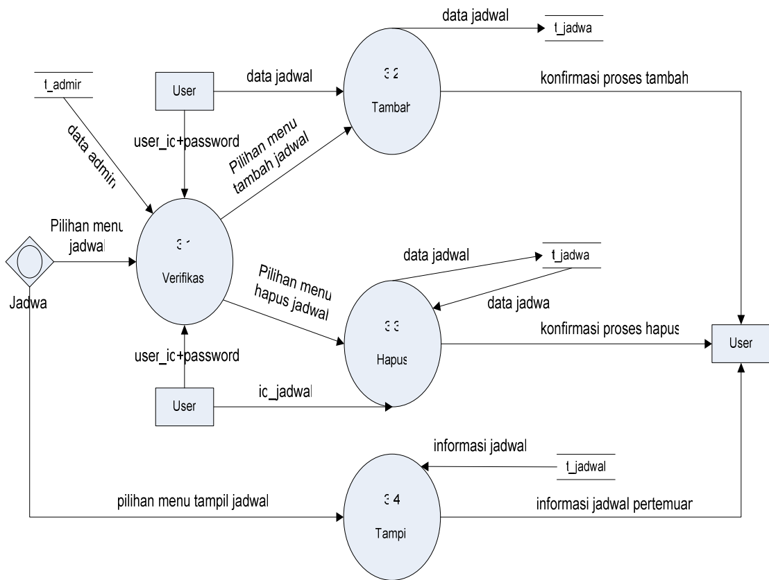
Gambar 3.1.1.2 Proses jadwal
