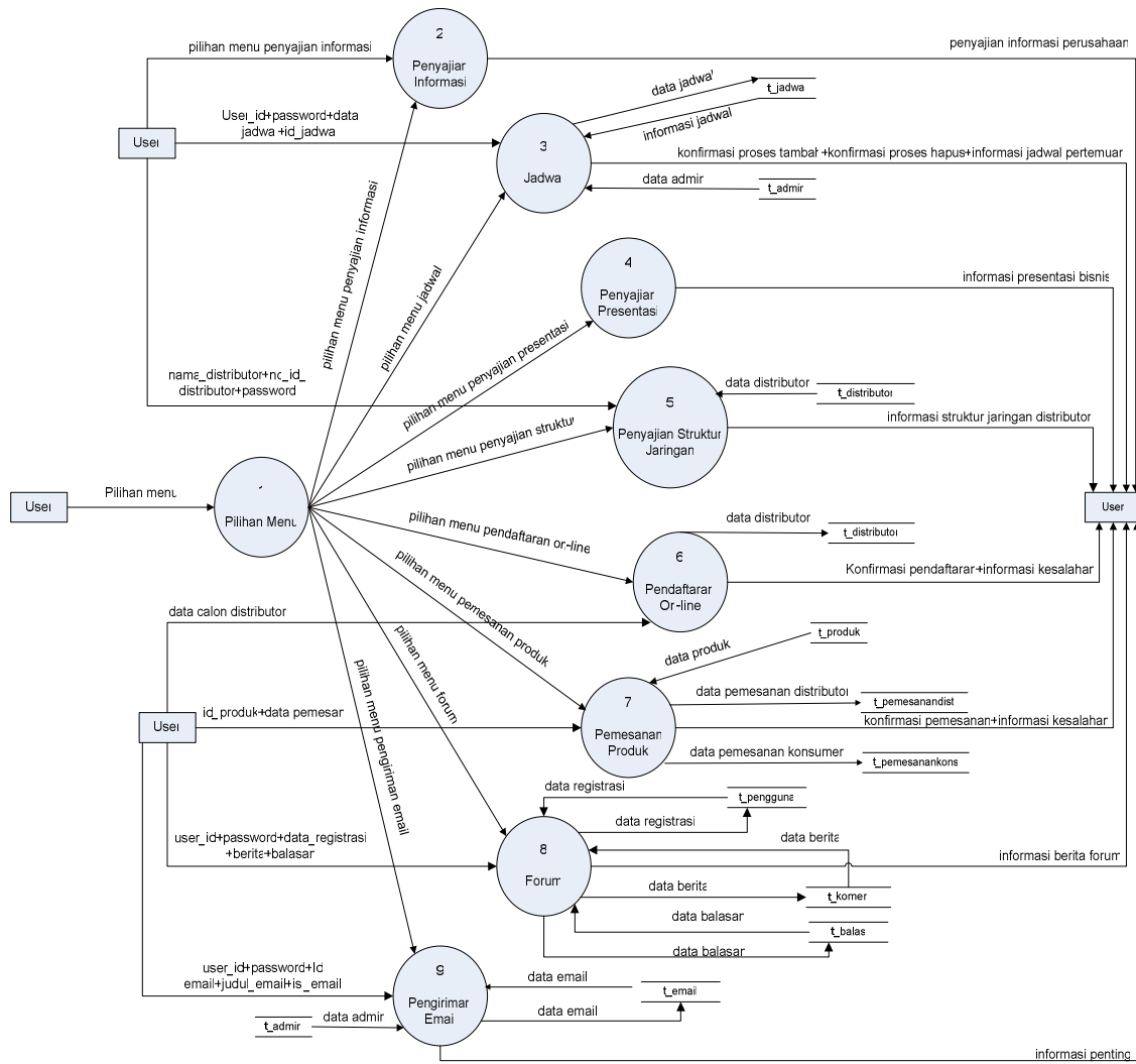
Gambar 3.1.1.1 DFD Level 1
