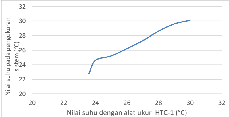
Gambar 15 Grafik Akuisisi data sensor DHT11
