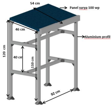
Gambar 4. Dudukan panel suryal
