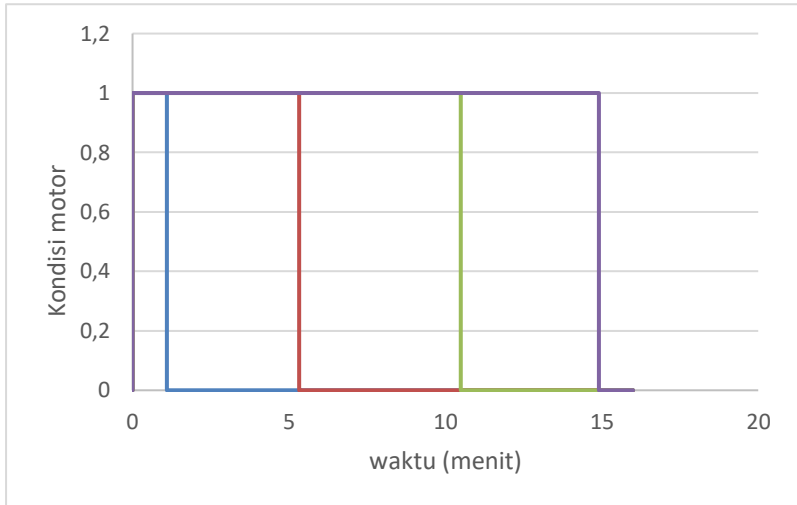
Gambar 20 Grafik Pengujian pada on off pompa
