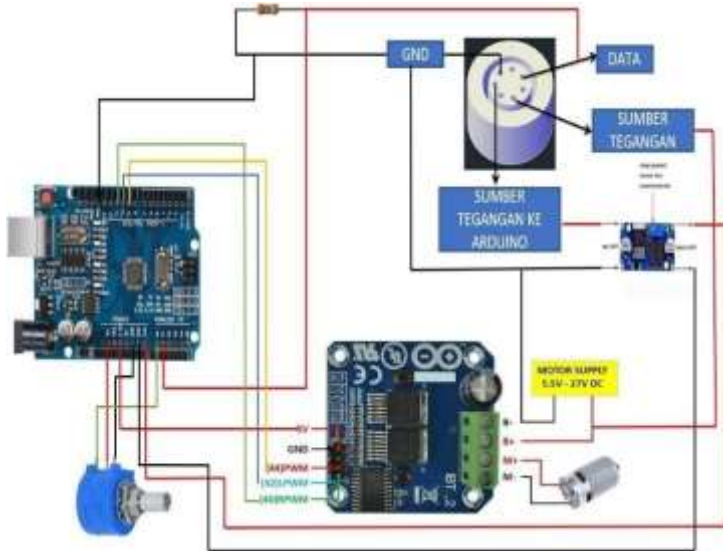
Gambar 2 Desain Elektrikal
