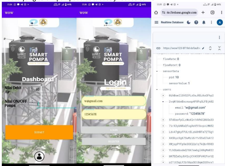
Gambar 18. Pengujian Aplikasi
