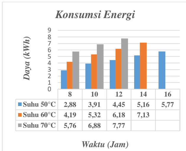
Gambar 7 Grafik Pengaruh Suhu dan Waktu Terhadap Daya
