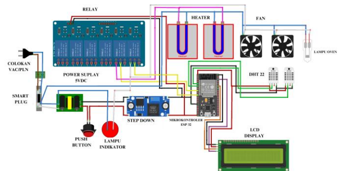
Gambar 4 Desain Elektrikal
