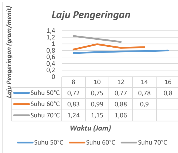
Gambar 9 Grafik laju Pengeringan
