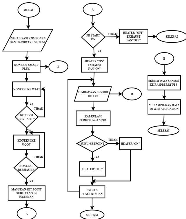
Gambar 5 Diagram Alir Sistem
