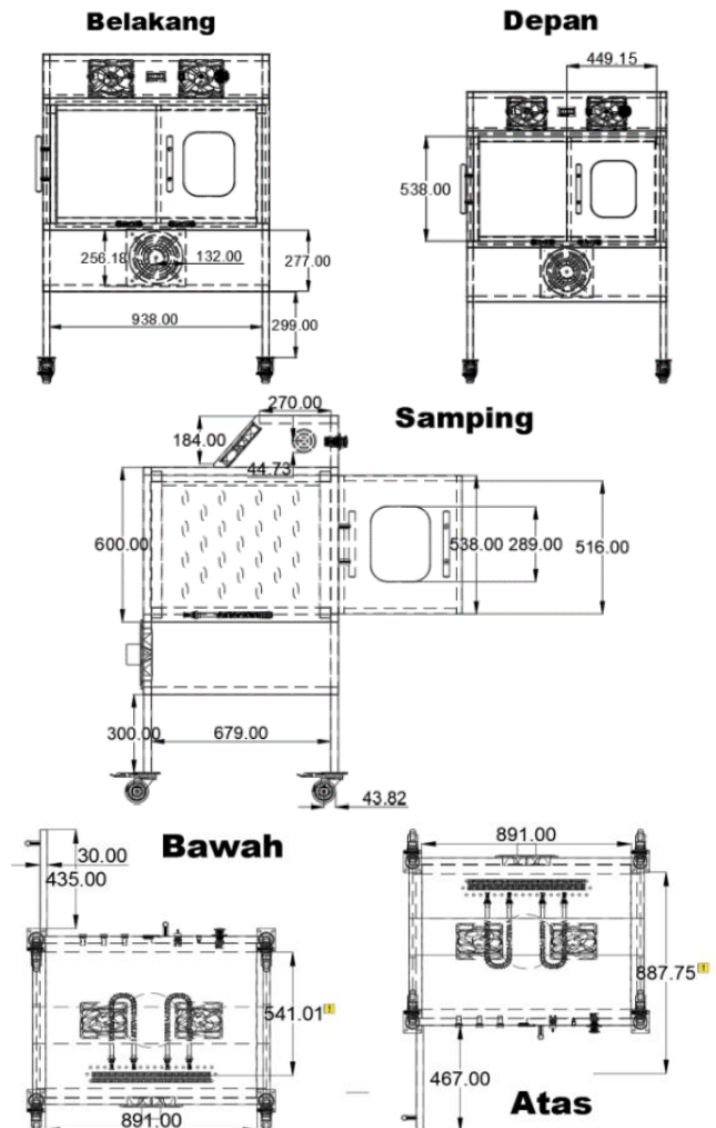
Gambar 3 Desain Mekanik
