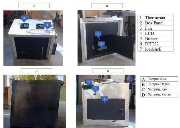
Gambar 2 Desain Mekanikal
