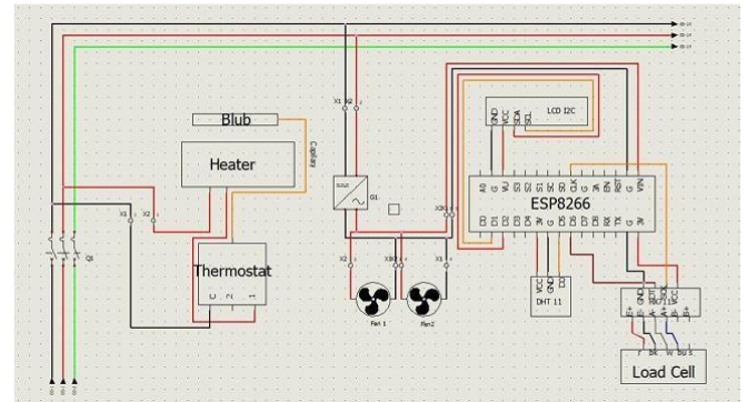
Gambar 1 Desain Elektrikal
