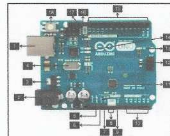
Gambar 1 Arduino Uno
