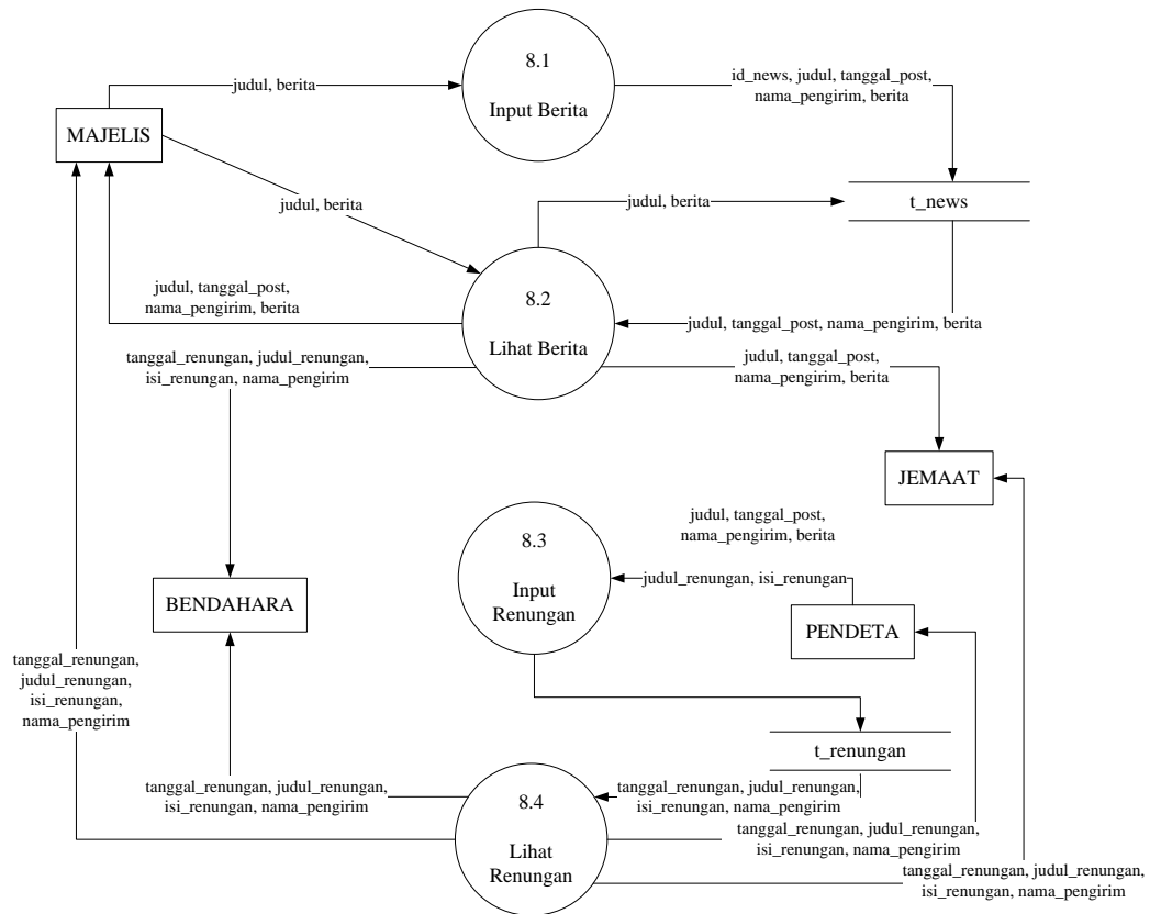
Gambar III-6.3.7 DFD Level 2 Proses 8 Berita/Renungan
