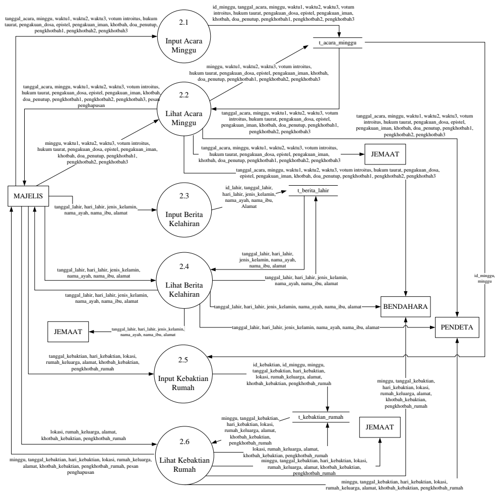
Gambar III-6.3.1 DFD Level 2 Proses 2 Informasi Acara Minggu
