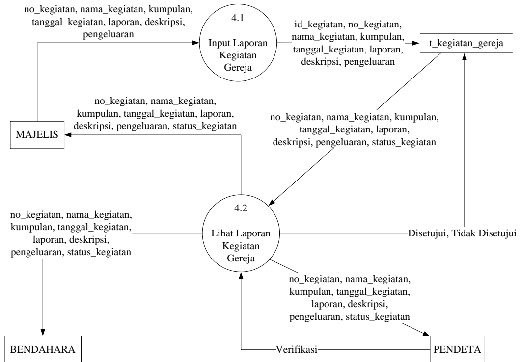
Gambar III-6.3.3 DFD Level 2 Proses 4 Pelaporan Kegiatan Gereja
