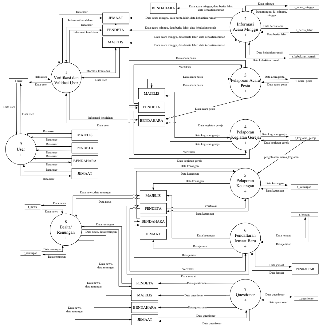
Gambar III-6.2 DFD Level 1
