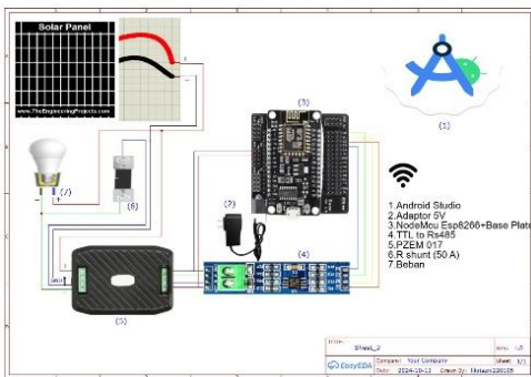
Gambar 4. Desain Elektrikal Sistem Monitoring
