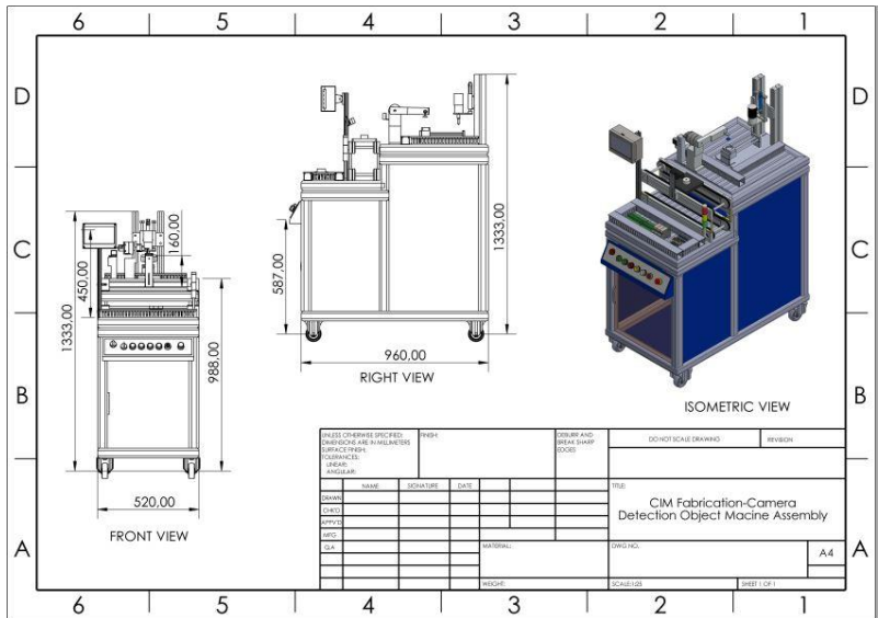
Gambar 25. Dimensi mesin
