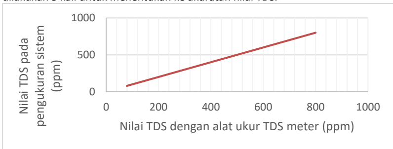
Gambar 18 Grafik Akuisisi data sensor TDS
