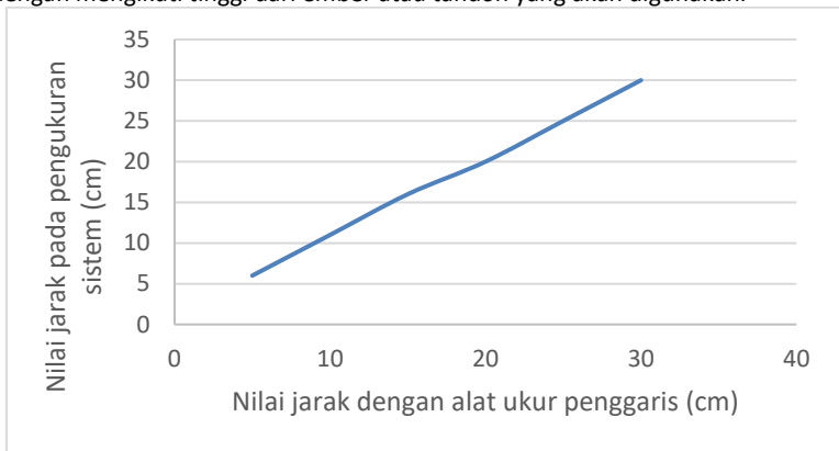
Gambar 16 Grafik Akuisisi data sensor HC-SR04t
