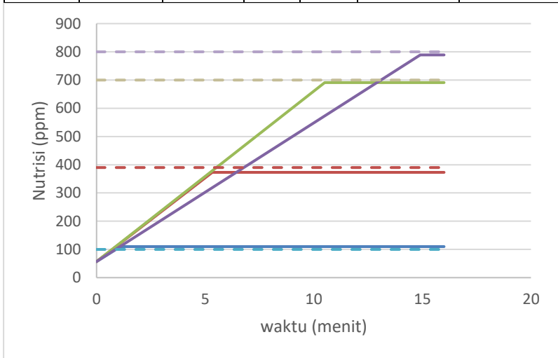
Gambar 19 Grafik Pengujian controlling
