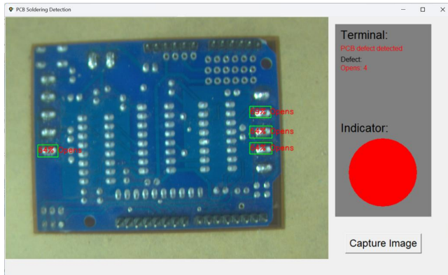
Gambar 11. Hasil deteksi sampel PCB yang REJECT/FAIL.
