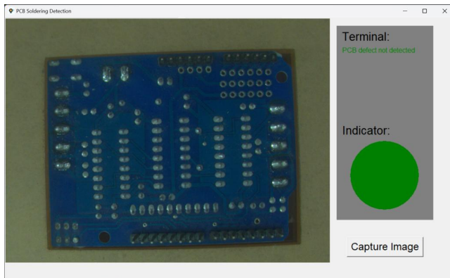
Gambar 12. Hasil deteksi sampel PCB yang GOOD/PASS.
