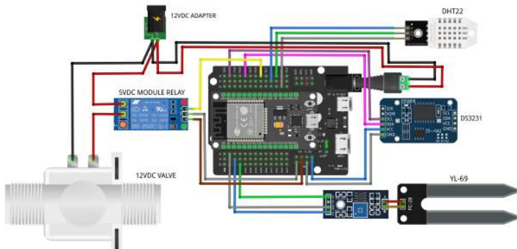
Gambar 4: Rangkaian elektrikal sistem
