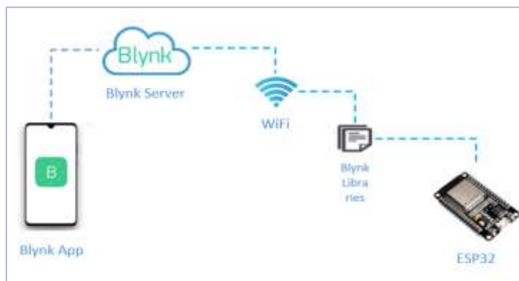
Gambar 8: Diagram topologi sistem komunikasi IoT aplikasi Blynk dan ESP32
