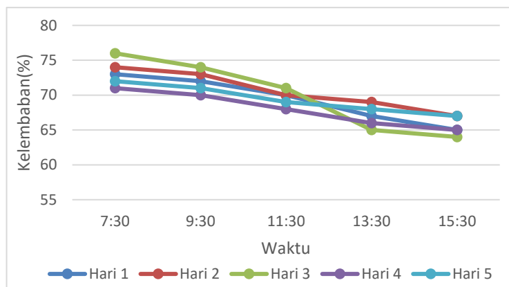
Gambar 11: Grafik perubahan kondisi kelembaban tanah
