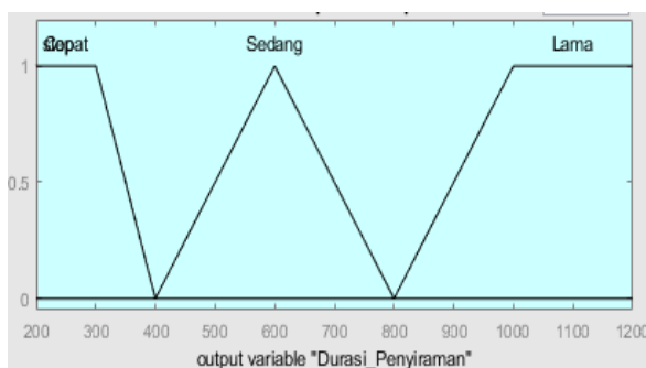
Gambar 7: Membership function output durasi penyiraman
