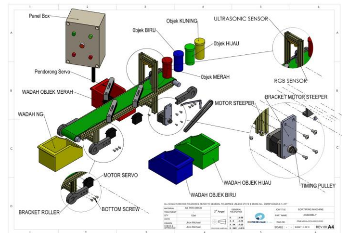
Gambar 5. Desain Mekanikal
