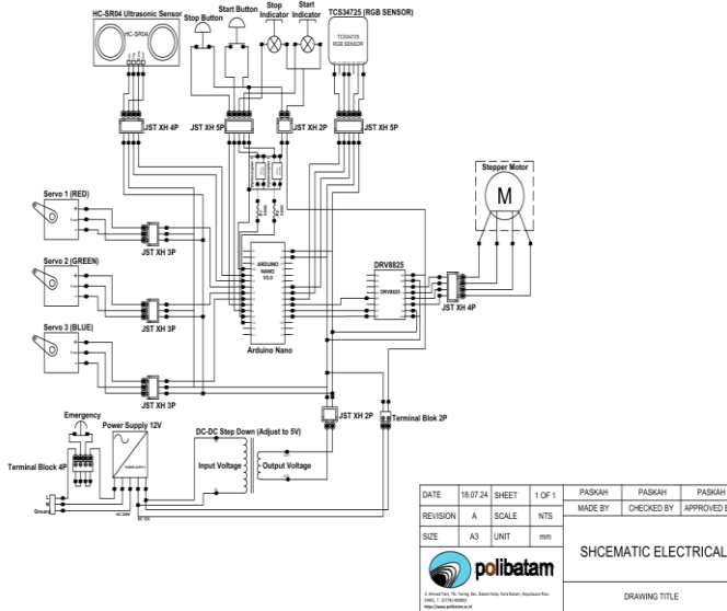
Gambar 6. Wiring Elektrikal
