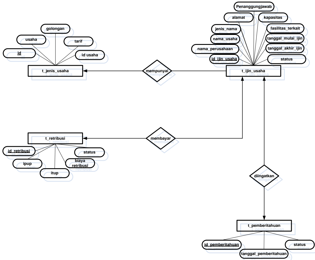
Gambar III.6 ER Diagram Sistem Informasi Masa Ijin Usaha Kepariwisata Kota Batam
